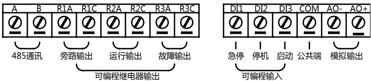
(上图标注的端子功能仅为默认设定值，实际功能可通过参数设定进行变更)
